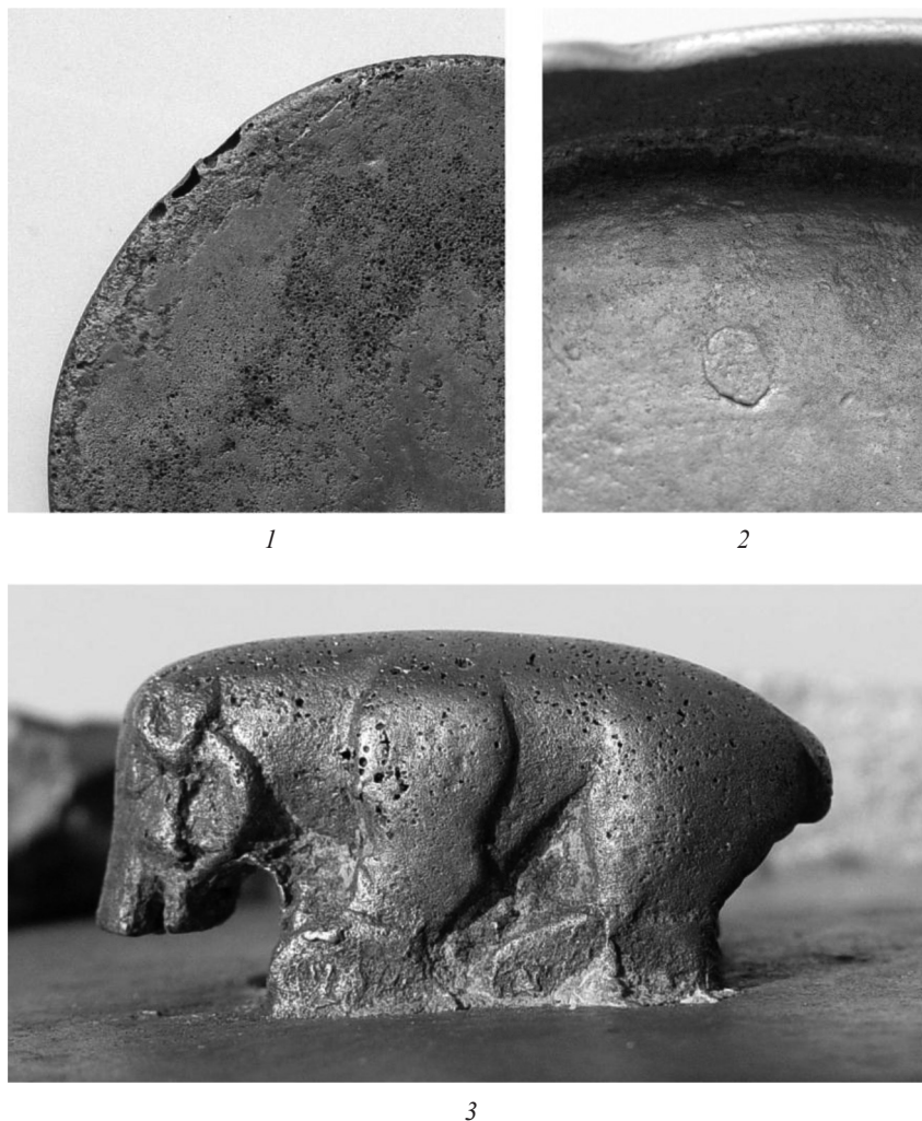
Рис. 2. Детали бронзового зеркала (могильник Бирлик, к. 29): 1 – лицевая сторона. Сварочный шов между двумя порциями залитого металла; 2 – расклепанный наплыв металла на оборотной стороне зеркала; 3 – фигура животного в профиль с залитым металлом промежутком между ног (литейный брак). Фото Е.А. Шаблавиной
