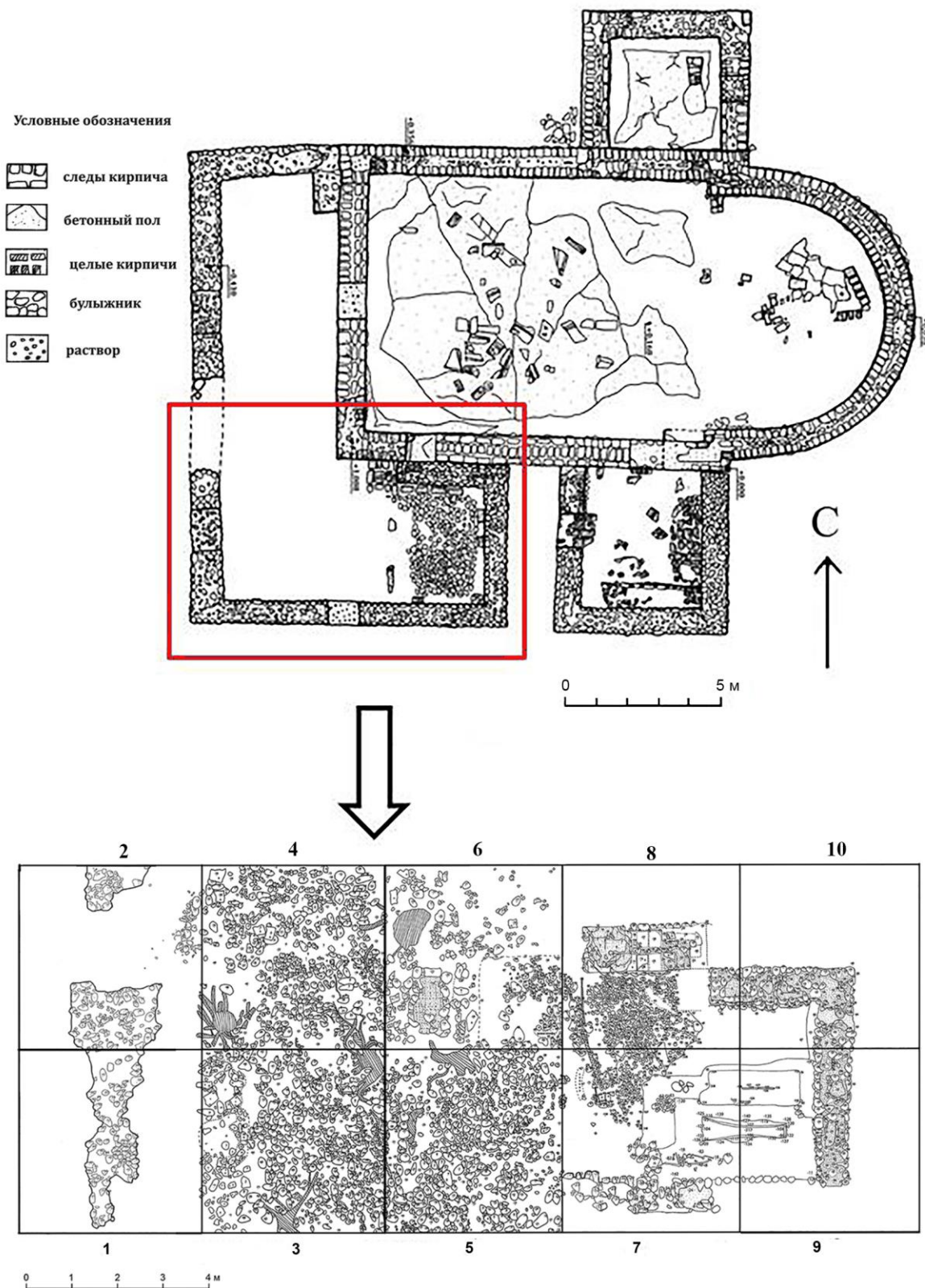
Рис. 2. Храм на городище Гиенос: общий план (А) и план западного раскопа (Б)
