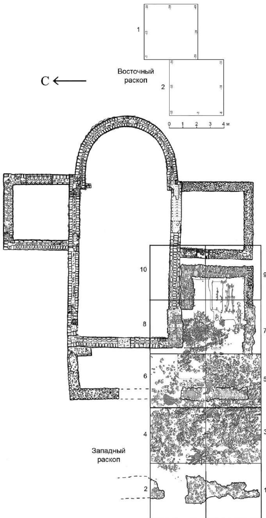
План храма на городище Гиенос, Западного и Восточного раскопов
